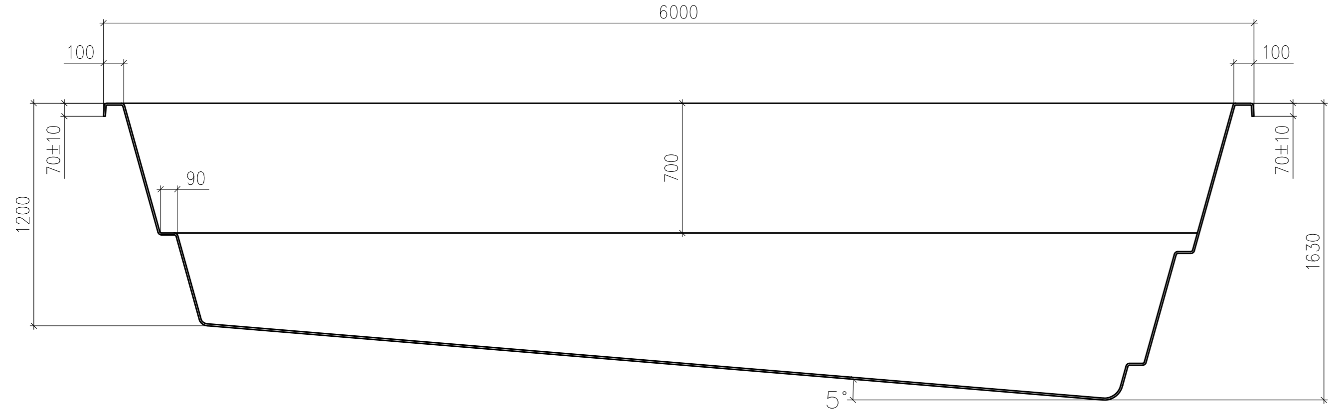
Разрез 1 - 1
